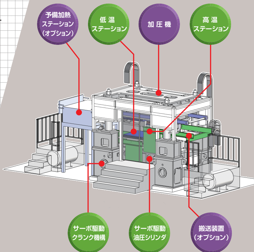
UFHS2500 CFRTP成形機
