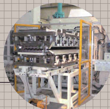
6Hi、21本ワークロール
